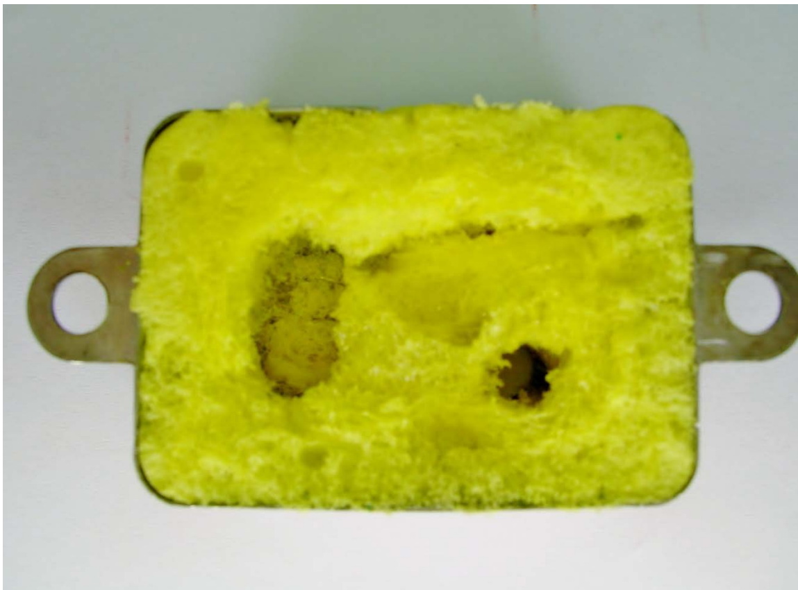
35. The LO shield prep.
